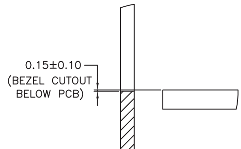
DETAIL K 2:1
